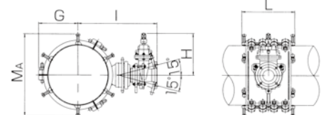
呼び径450×75～900×200
