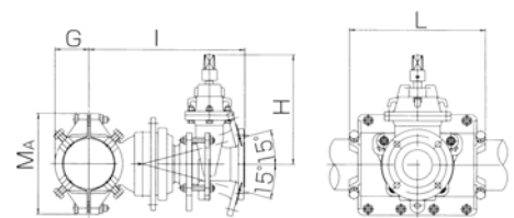
呼び径450×75～900×200
