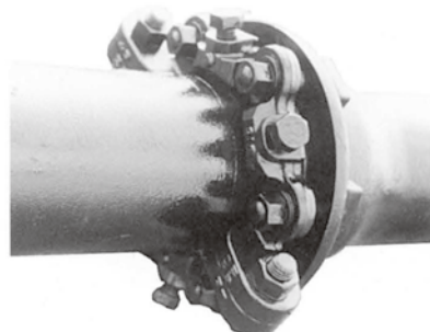
短ボルトナットK形パッキン付
