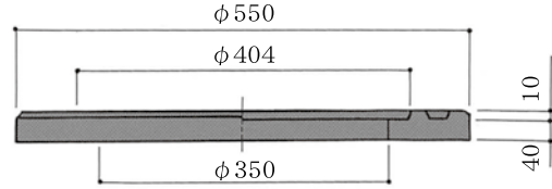
NHVO-25-40S(底板)
