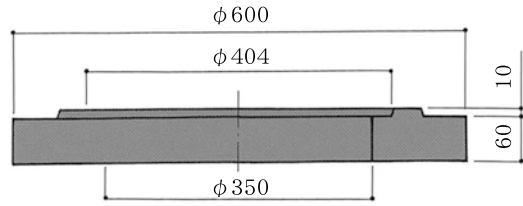
NHVO-25-60S(底板)
