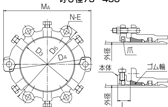
呼び径75～450
