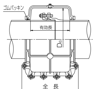
呼び径350～700
