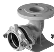
チーズF型 うずまき式
