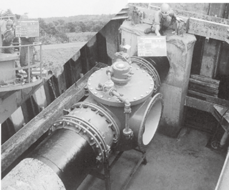
稚内市水道部 SP \phi 900 インサートバルブT型
