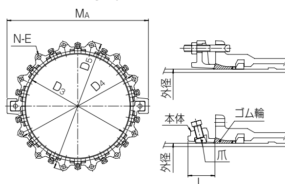
呼び径500～1000
