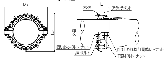
呼び径300～450
