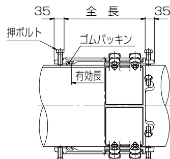
呼び径400～1000
