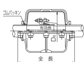
呼び径75～300
