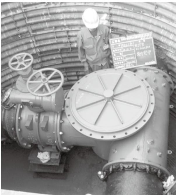
札幌市水道局 \phi 700 \times \phi 700 HC工法
