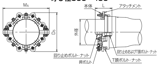
呼び径300～450
