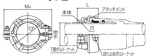
呼び径75～250
