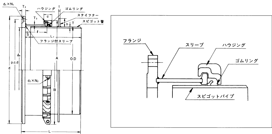
フランジアダプター寸法 ※価格はP459に掲載しています。 材質：SS400フランジ7.5K、SUS製も製作可能です。 単位:mm
