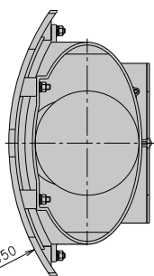
1号、2号、3号共通寸法
