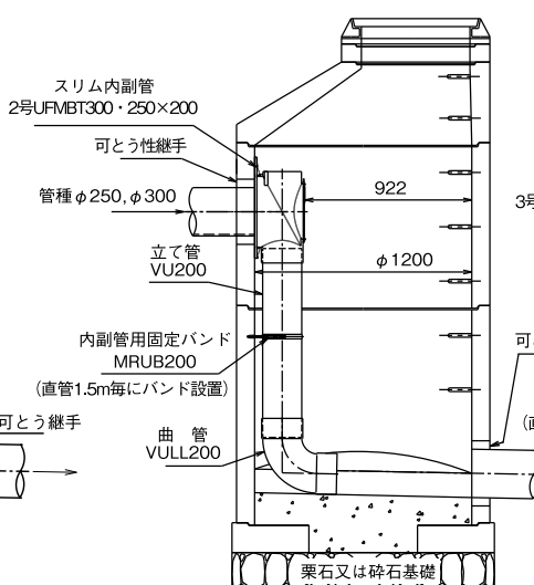
断面図
